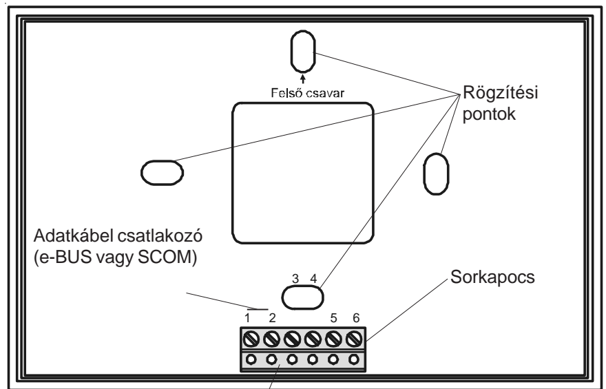
Tűs csatlakozó a szabályozóhoz
